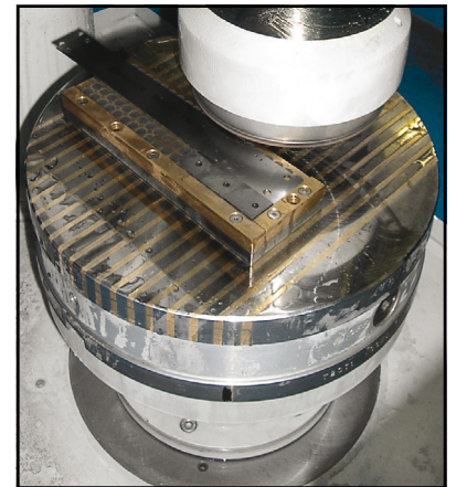
Piano magnetico a campo aperto オープン・フィールド・マグネット式作業面 Magnettisch für HM Werkstücke
