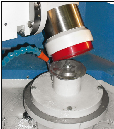
Flangia per tavola rotante 標準回転テーブル用フランジ Flansch für Standard-Drehtisch
